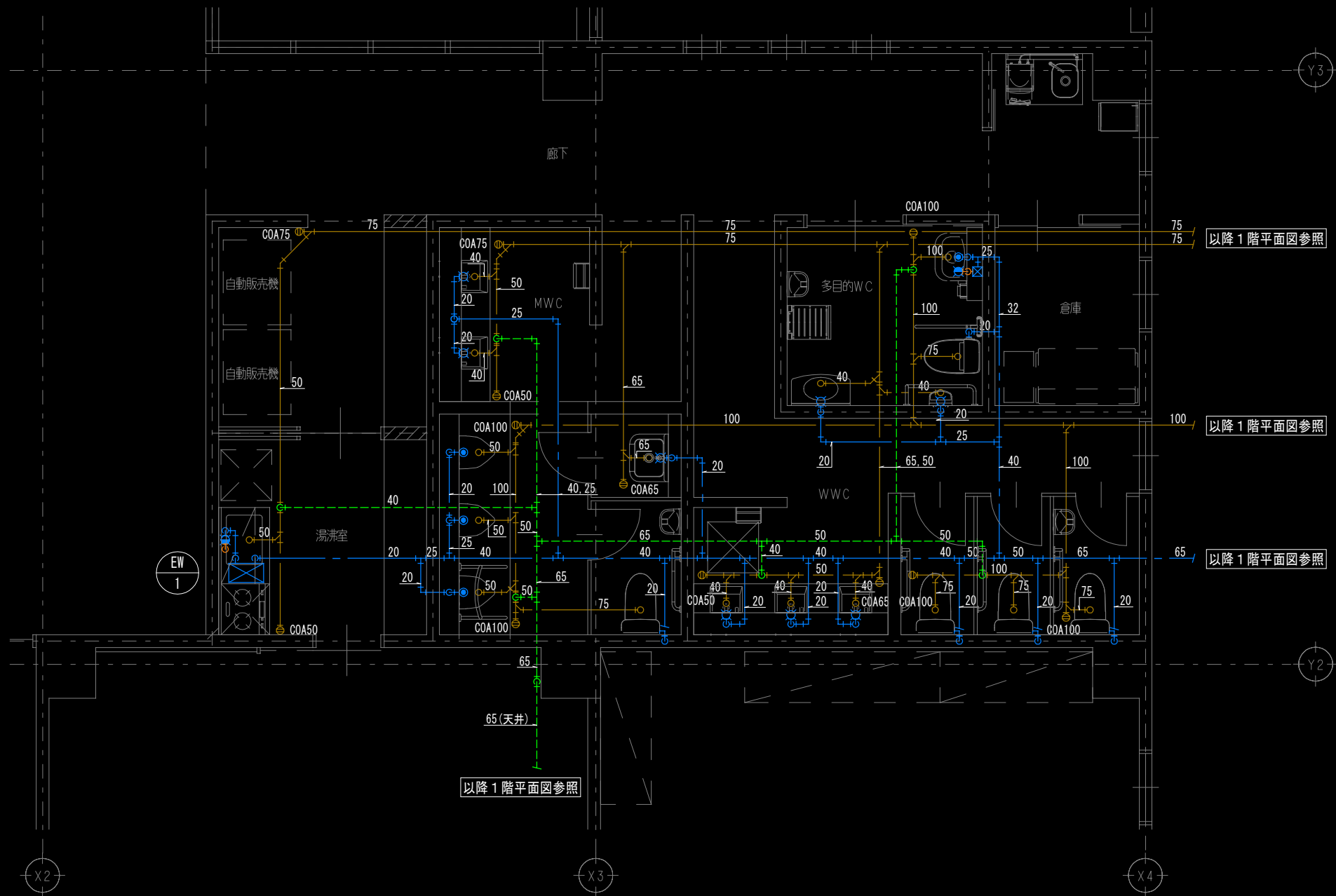
W C 廻り平面詳細図
