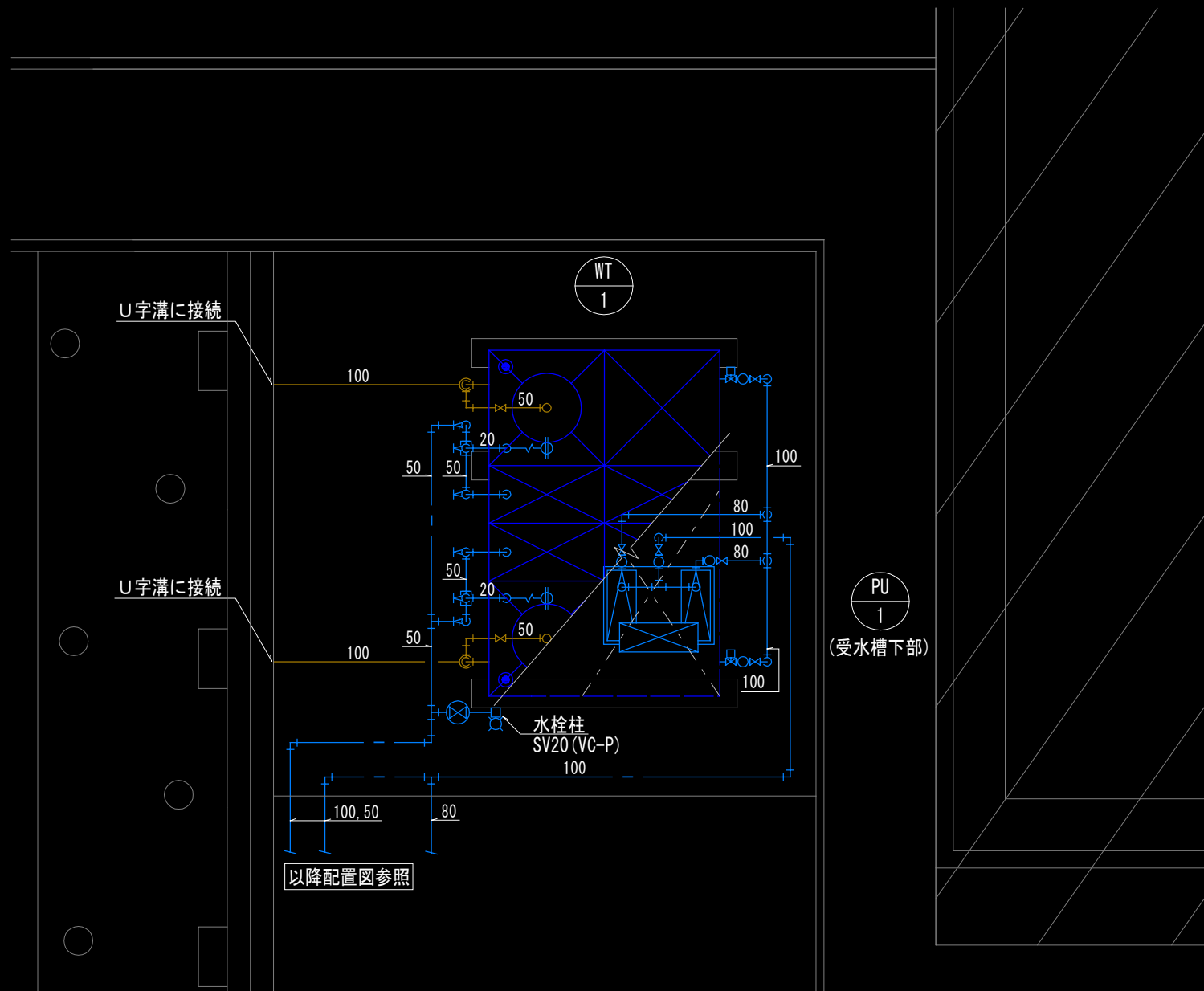
受水槽・給水ポンプ廻り詳細図
