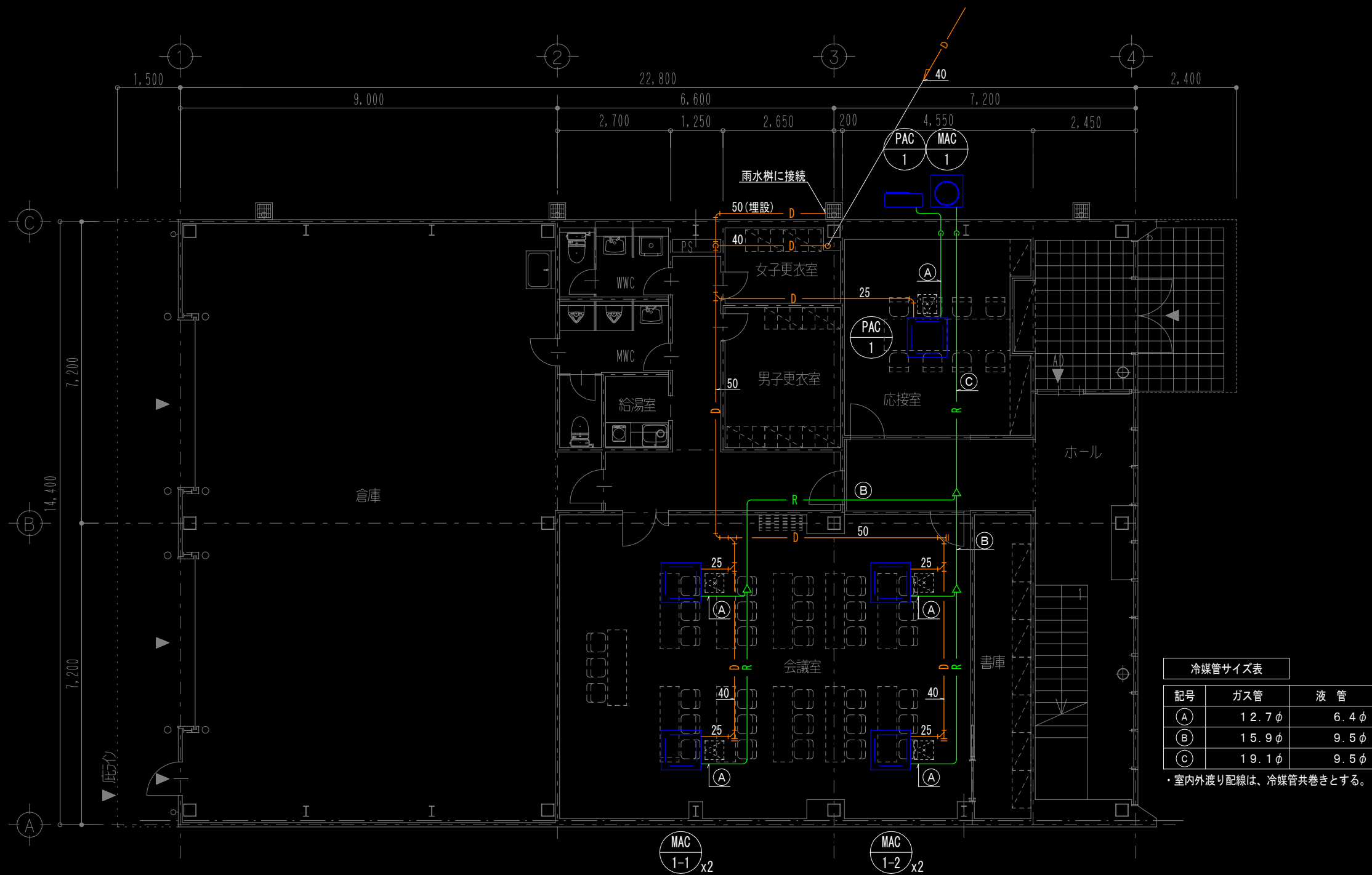
空調設備 配管平面図
